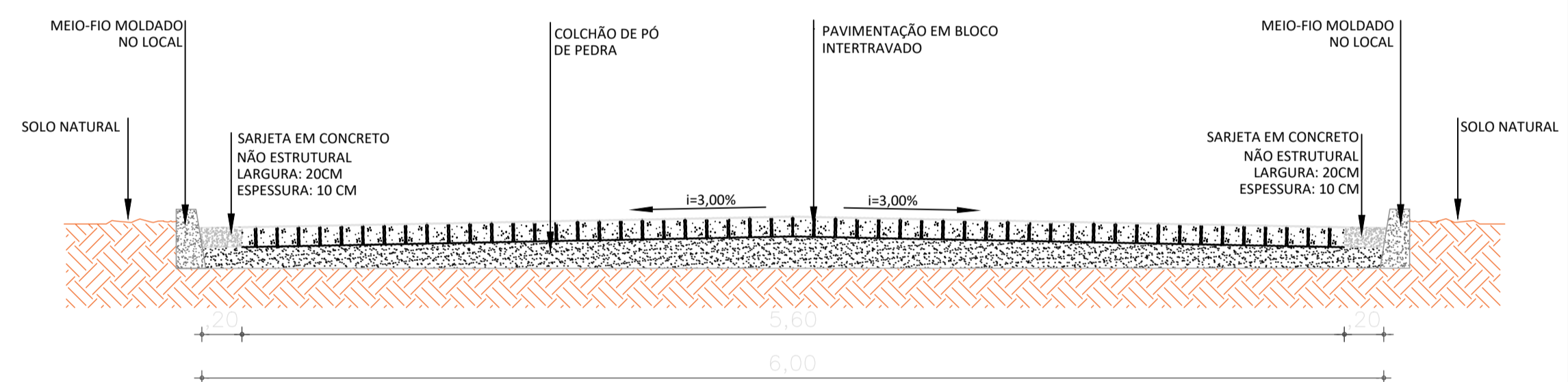
03 CORTE TRANSVERSAL
